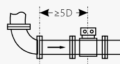
90°弯头
