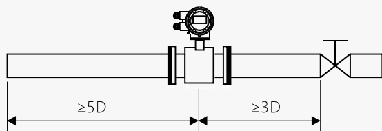
阀门在传感器下游的安装
