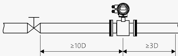
阀门在传感器上游的安装
