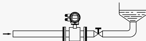
传感器下游有背压的安装
