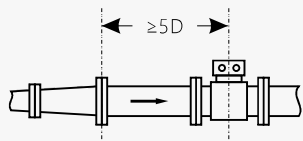
扩张管
