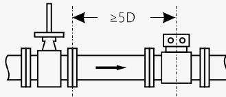
全开的闸阀
