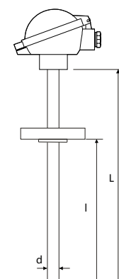
固定法兰形式
