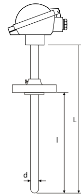
活动法兰形式
